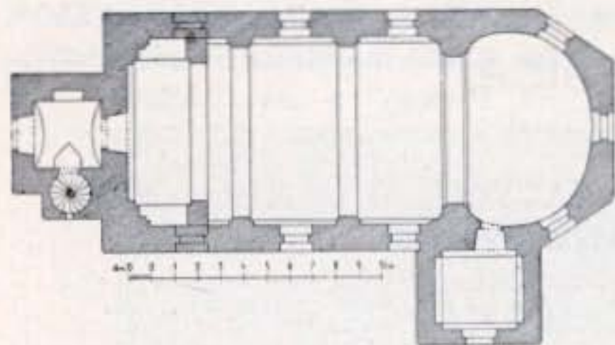
Obr. 361. Tepléžovice, Půdorys kostela.
